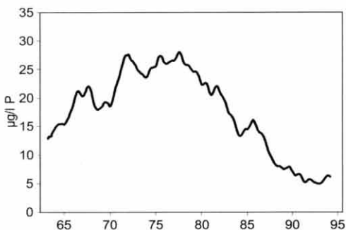
Abb. 3. Entwicklung des Gesamt-Phosphorgehaltes im Vierwaldstättersee 1964–1994 (aus Bühler & Ambühl 1996). – Total Phosphorus content in Vierwaldstättersee 1964–1994.
